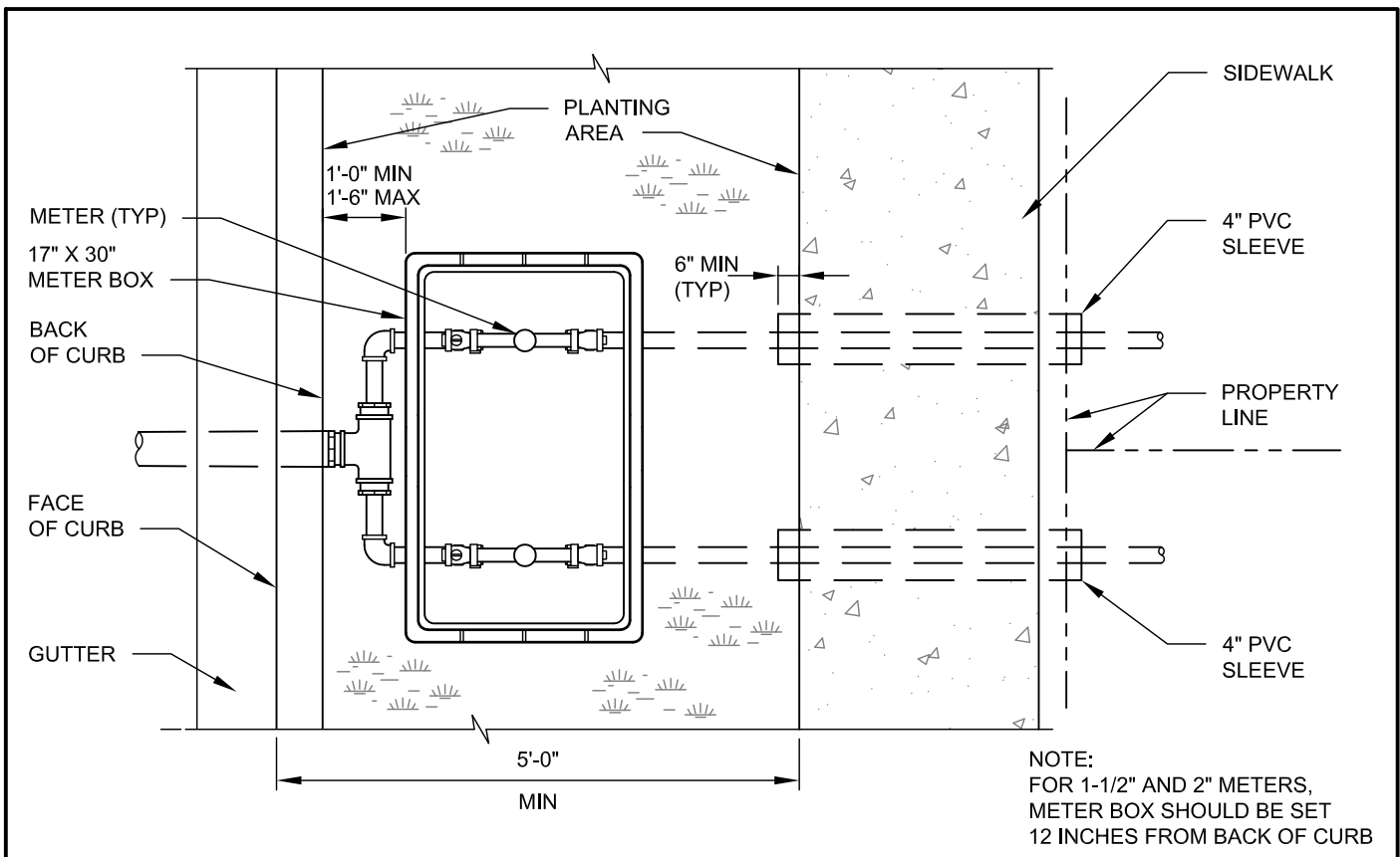
METER BOXES NTS
